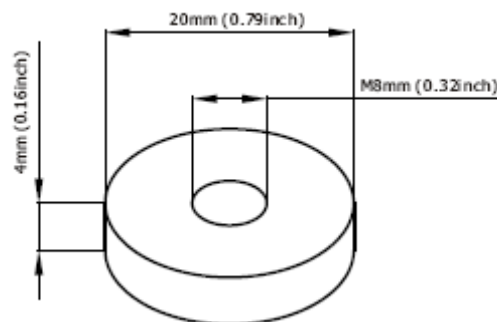
Dimensiuni bornă
